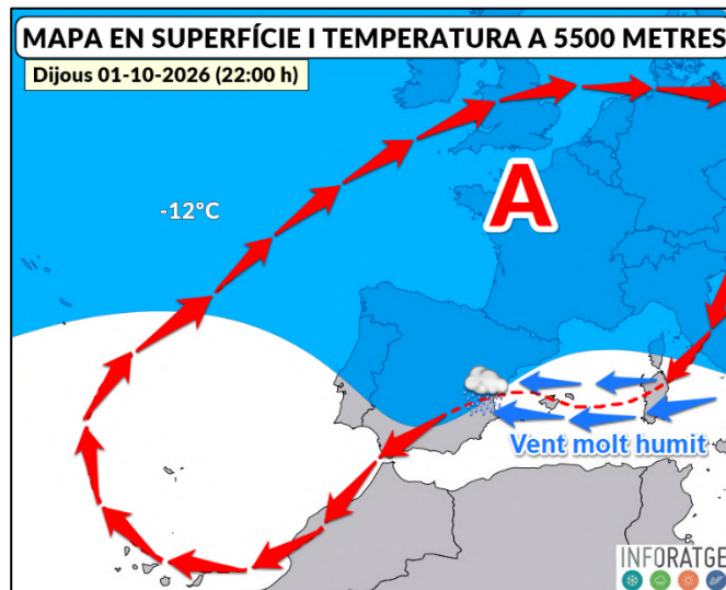
Mapa de la temperatura a 5500 metres y situación en superficie el 01-10-2026 a las 22:00 h (Fuente: Inforatge)
