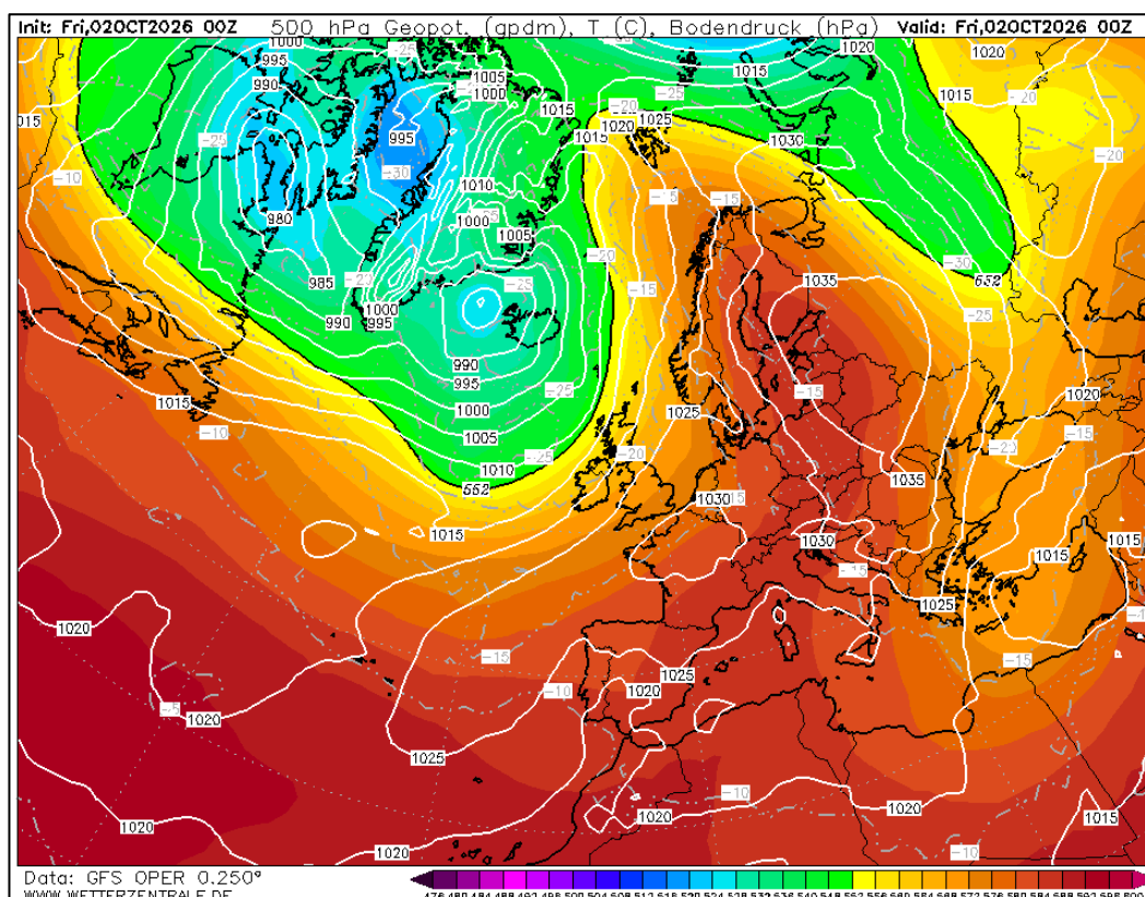
Situación sinóptica del 02-10-2026 (00Z). Geopotencial a 500 hPa y mapa de superficie.
